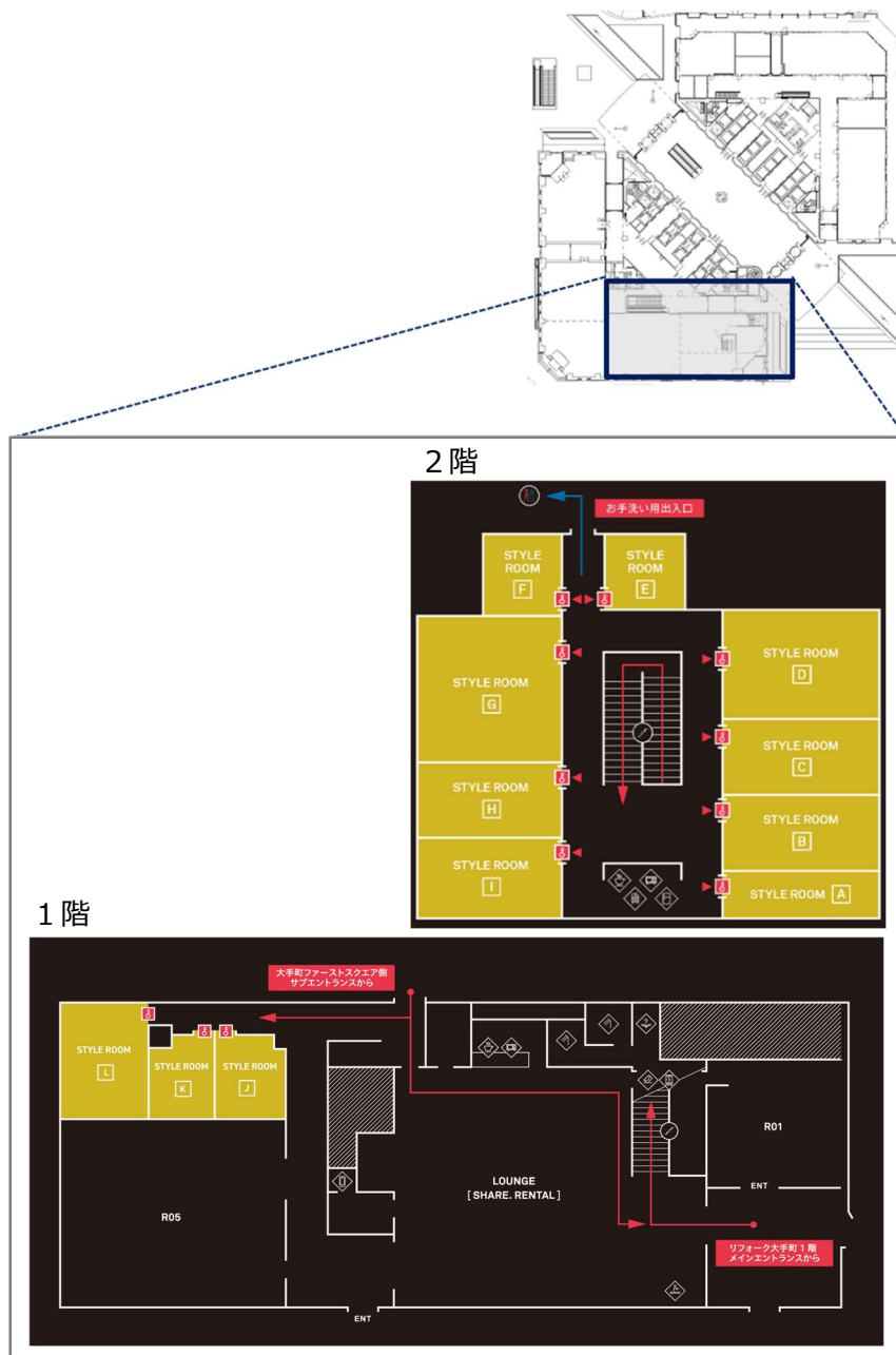
大手町ファーストスクエア ウェストタワー1・2階 平面図
